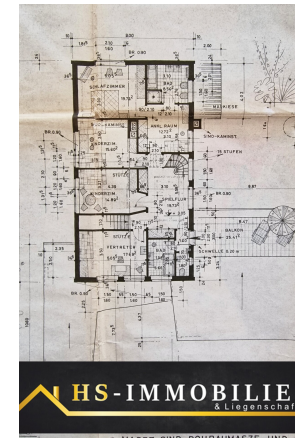
Plan I. OG
