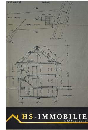
Schnitt
